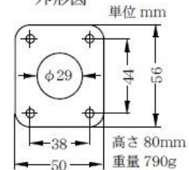
外形図
